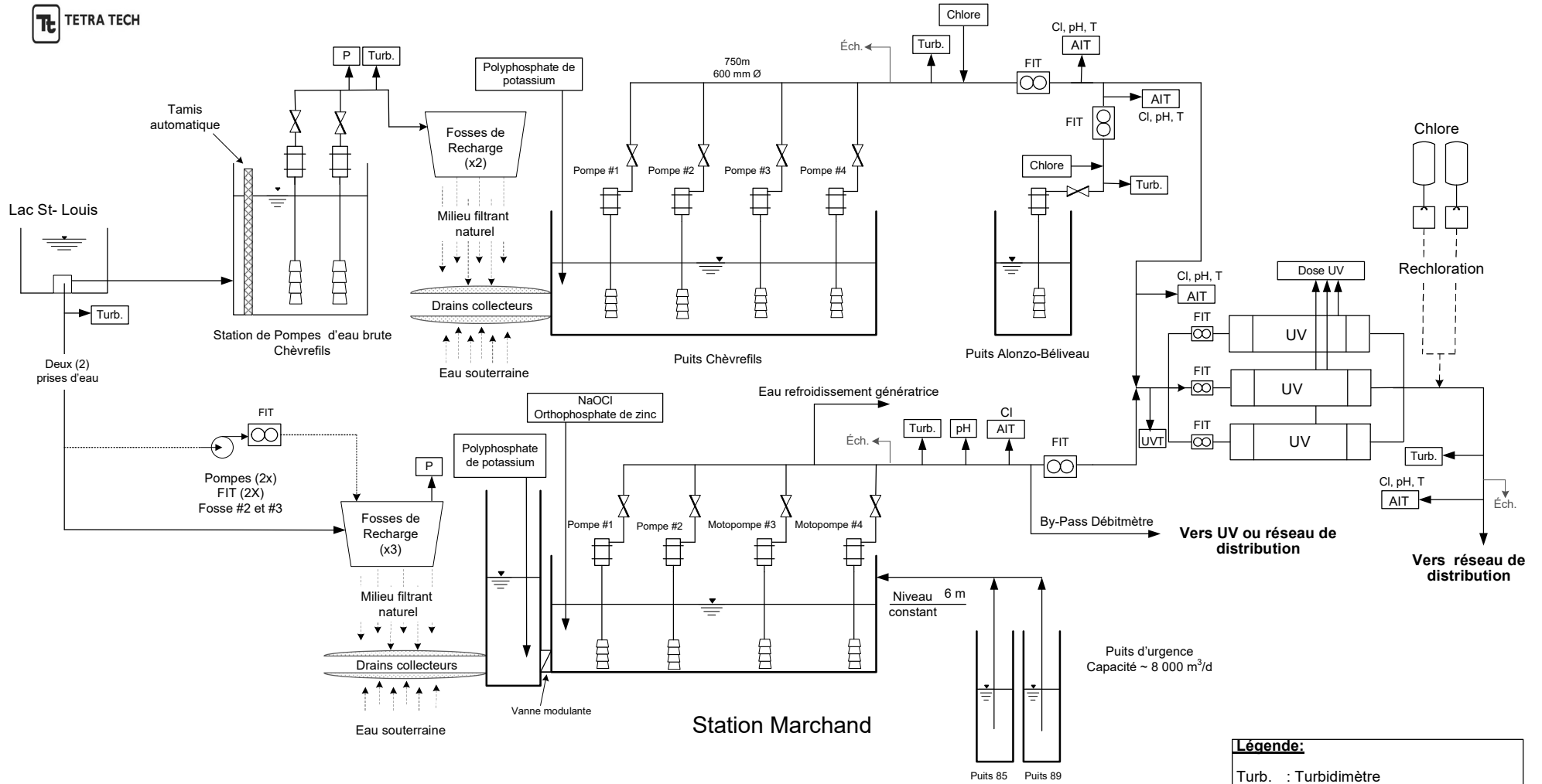
Figure 1 : Schéma de procédé des installation de production d'eau potable - Ville de Châteauguay
